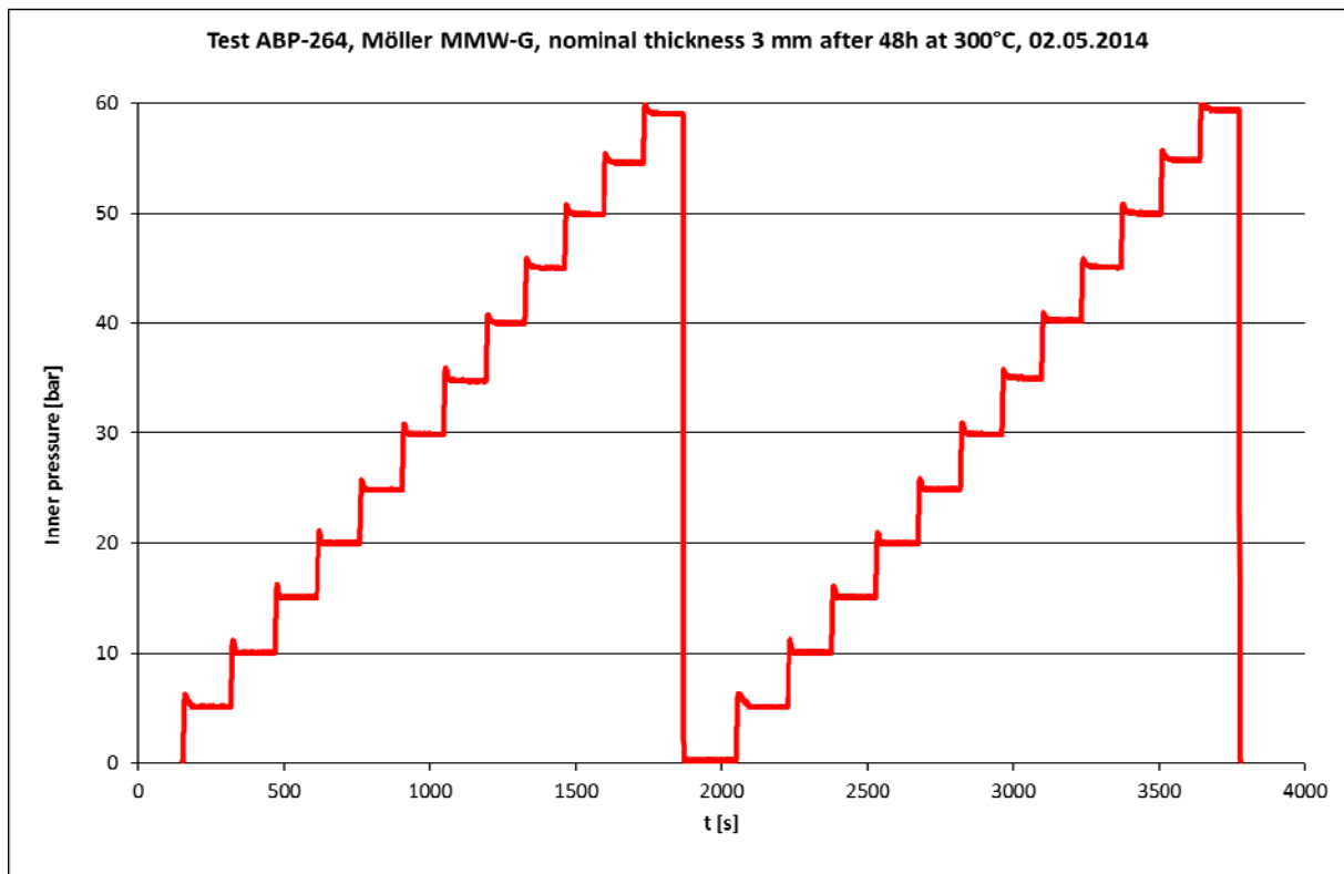
Diagramm 1: Ausblastsicherheitstest
