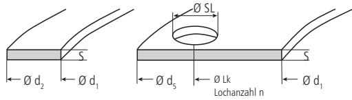
Maße von Flachdichtungen nach DIN 86072-1 für Flansche nach DIN 86044-1 (schwere Ausführung), Dicke s = 2 mm
